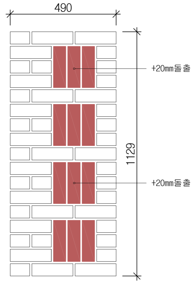
A우측면도
