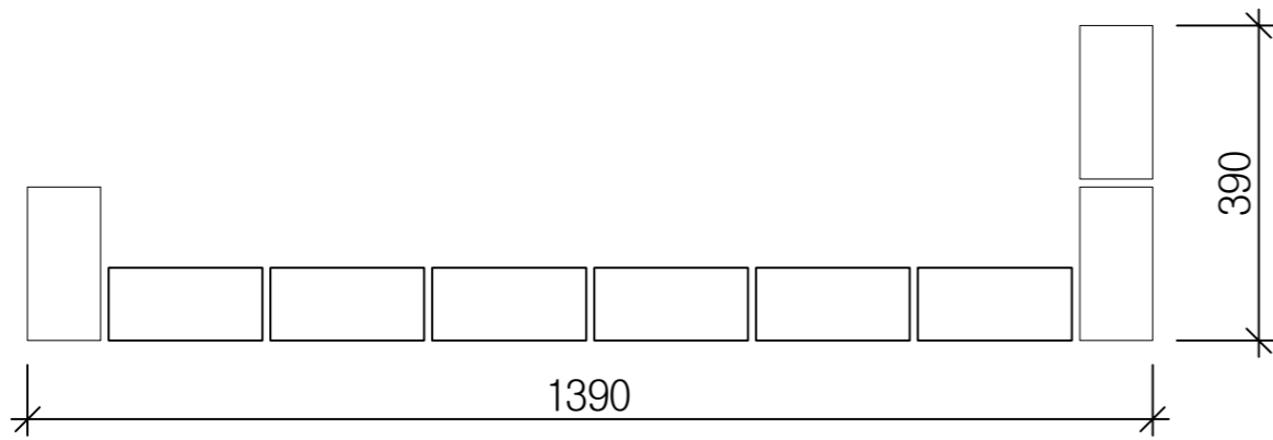
○ 평면도
