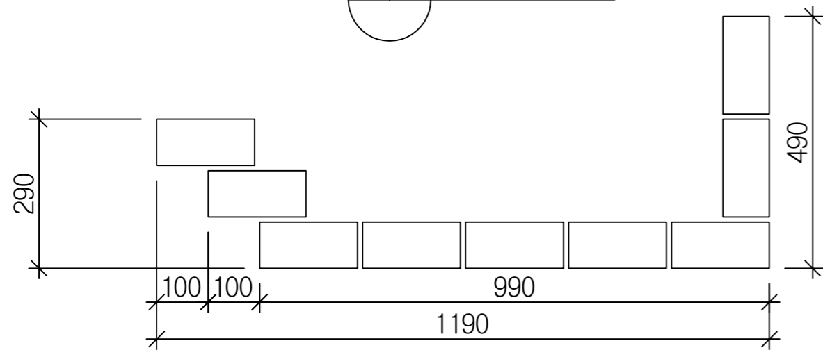
평면도
