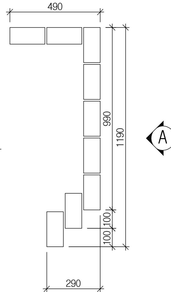
1켜 평면도
