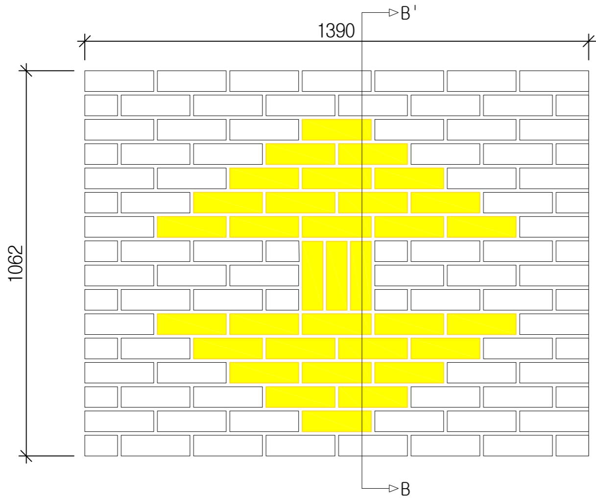
○ B정면도
