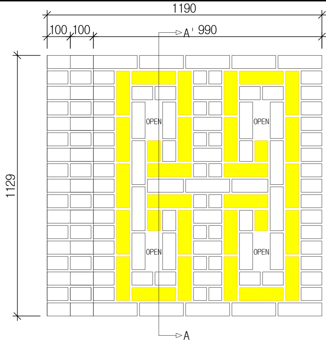
A정면도
